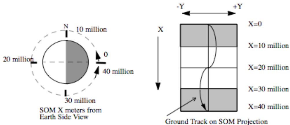
Figure A-4 Attributes of SOM coordinates
