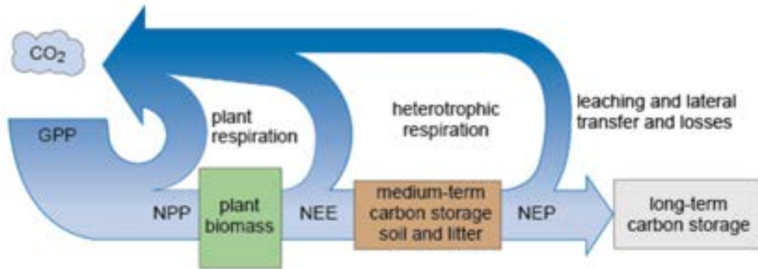
Figura 2.2.21 La producción neta del ecosistema (NEP por sus siglas en inglés) es igual al intercambio neto del ecosistema (NEE por sus siglas en inglés) menos las pérdidas por lixiviación incluyendo pérdidas o ganancias por transferencias laterales de carbono. NEP es equivalente a la cantidad de carbono acumulada en el material orgánico (vivo y muerto) durante el período estipulado (normalmente 1 año. complejo de evolución de oxígeno
